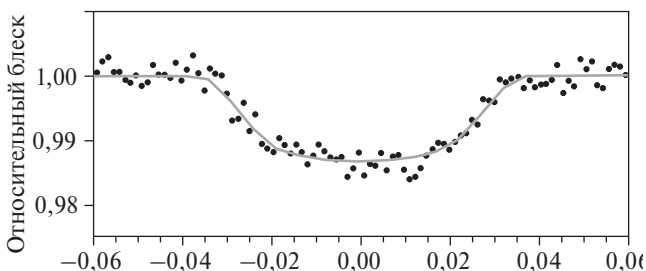
График кривой блеска транзита экзопланеты KPS-1b по диску родительской звезды UCAC4 775-030421, полученный на основе данных телескопа Т-100 Национальной обсерватории “Тюбитак” (Турция). Имеет характерную U-образную форму с продолжительным минимумом
