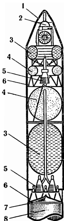
Рис. 18. Схема головного блока четырех-ступенчатой ракеты-носителя «Молния»:
