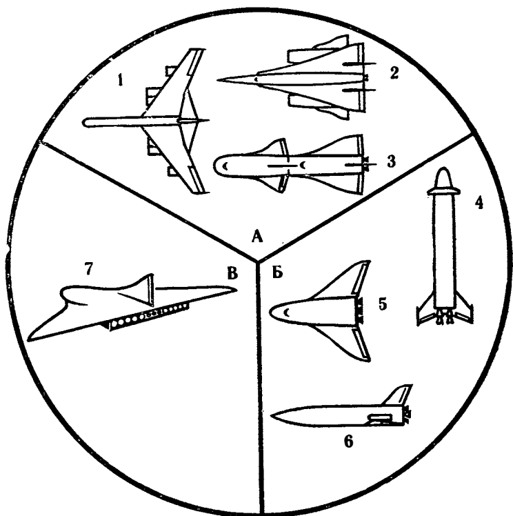
Р и с. 35. Возможные транспортные космические системы:
