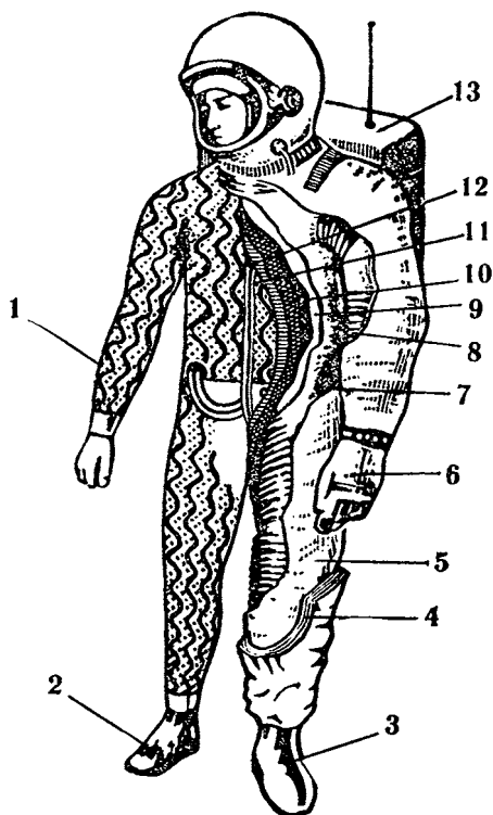
Рис. 45. Скафандр исследователя Луны:
