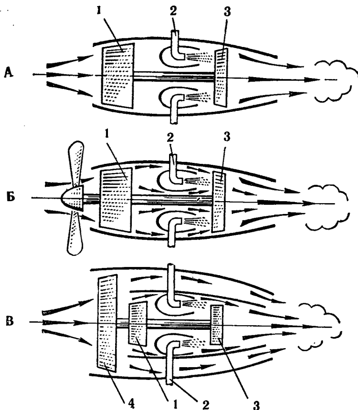
Рис. 31. Воздушно-реактивные двигатели.
