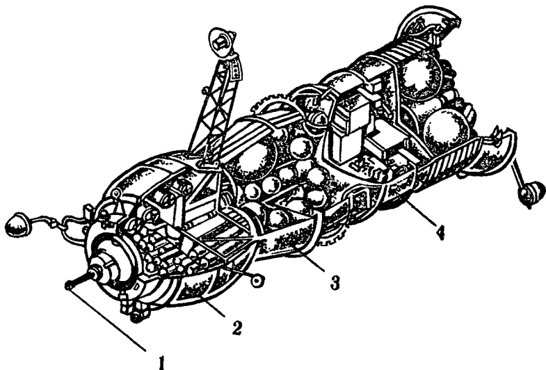
Р и с. 27. Космический корабль «Прогресс»:
