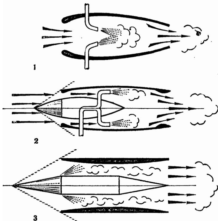
Р и с. 32. Схемы прямоточного воздушно-реактивного двигателя: 1 — дозвуковые и малые сверхзвуковые скорости полета — до 600 м/с; 2 — сверхзвуковая скорость полета — до 2 км/с; 3 — гиперзвуковая скорость полета — до 3 км/с
