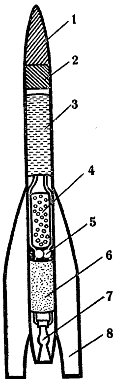
Рис. 10. Экспериментальная ракета ГИРД-10:
