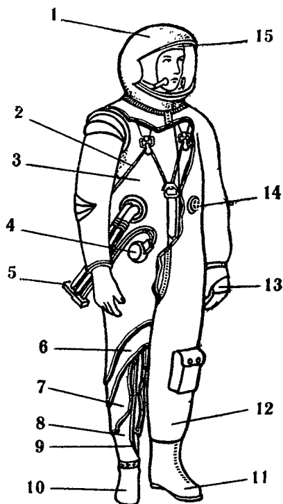
Рис. 23. Скафандр космонавта:
