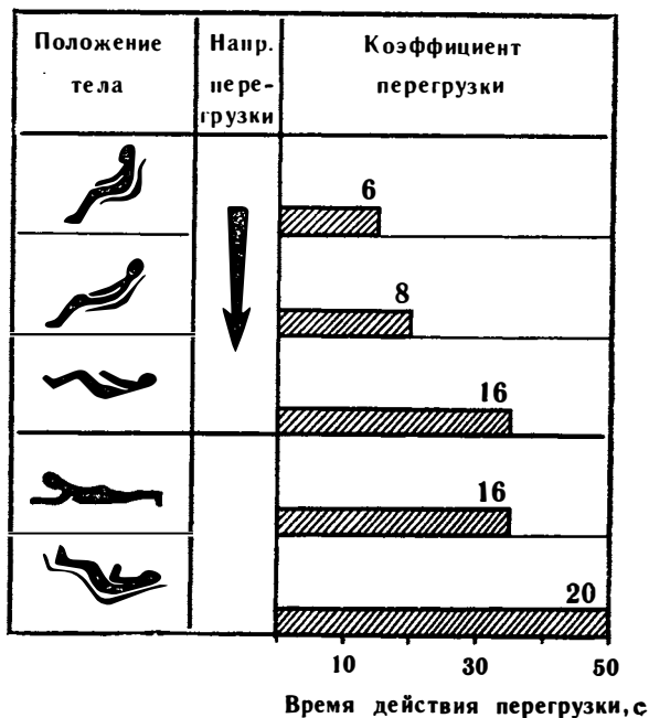
Рис. 4. Коэффициент переносимой перегрузки при определенном положении тела
