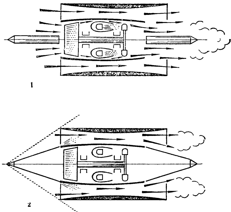
Рис. 33. Схема турбопрямоточного двигателя: 1 — работа по схеме турбореактивного двигателя; 2 — работа по схеме гиперзвукового прямоточного воздушно-реактивного двигателя
