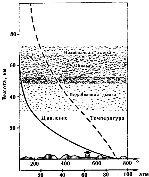
Р и с. 50. Атмосфера Венеры
