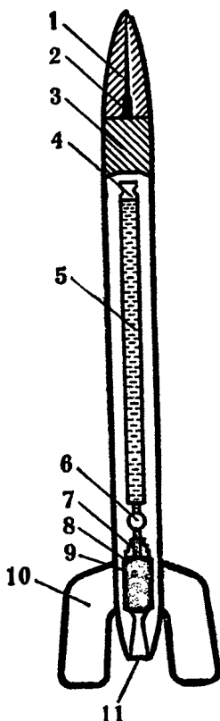
Рис. 10. Экспериментальная ракета ГИРД-10:
