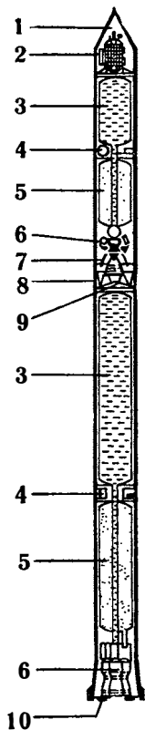
Рис. 20. Двухступенчатая ракета-носитель «Космос»:
