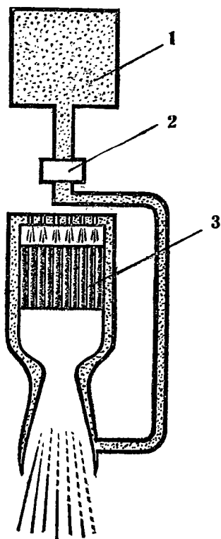
Рис. 16. Схема ядерного ракетного двигателя:
