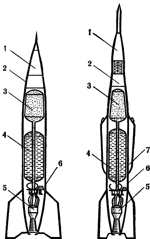
Рис. 12. Геофизические ракеты В-1А и В-1Е:
