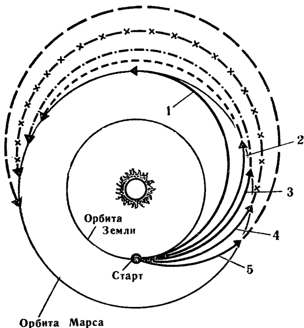
Рис. 48. Время полета к Марсу при различной начальной скорости отлета космического корабля с Земли
