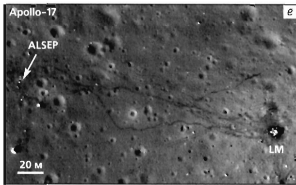
Рис.4. Снимки мест посадки КА «Аполлона-11, -12, -14-16 и -17», полученные камерами LROC NAC с борта КА «Lunar Reconnaissance Orbiter». Эксперименты: ALSEP — Apollo Lunar Surface Experiments Package, PSEP — Passive Seismic Experiment, LRRR — Lunar Laser Ranging Experiment.
