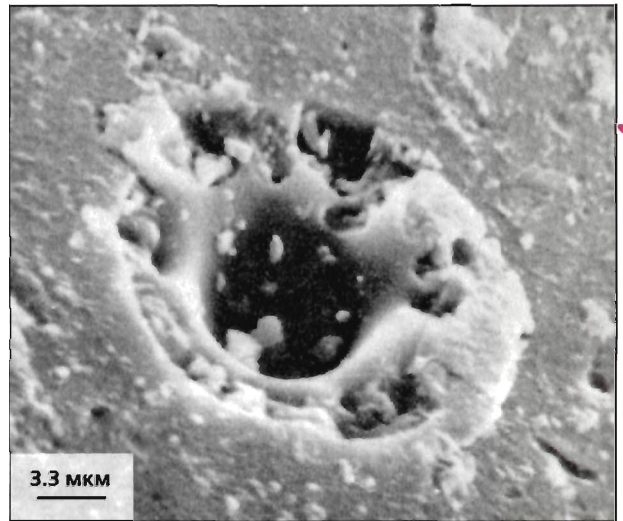
Рис.3. Шарик ударного расплава из грунта, доставленного одним из «Аполлонов» (слева) и микрократер на стеклянном шарике из коллекции «Луны-16». Изображения получены методом сканирующей электронной микроскопии.
