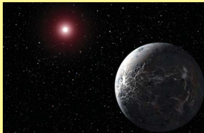
OGLE-2005-BLG-390Lb в представлении художника
