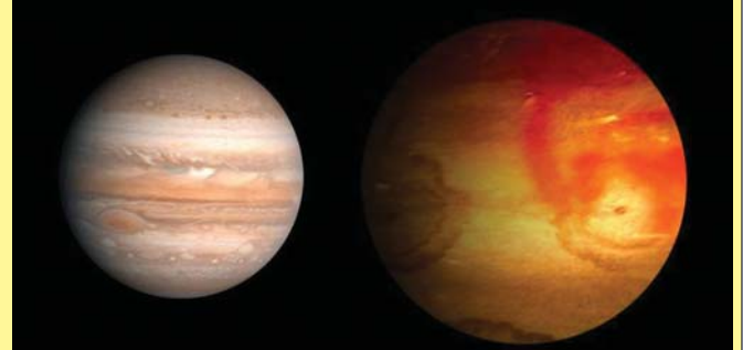
Художественное изображение HAT-P-7b в сравнении с Юпитером
