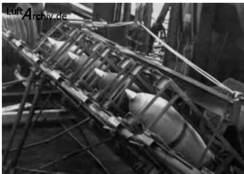
Первые ракеты морского базирования на борту немецкой ПЛ
