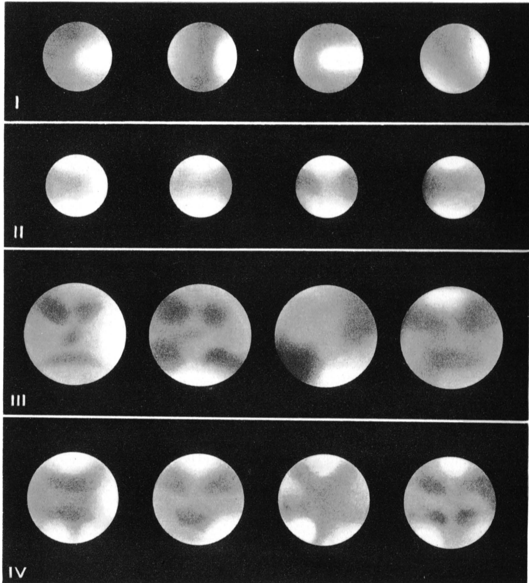
ASPECTS DES SATELLITES DE JUPITER D'APRÈS LES OBSERVATIONS EFFECTUÉES AU PIC DU MIDI PAR LYOT, CAMICHEL ET GENTILI (1941-1943).
