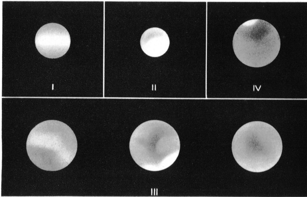
ASPECTS DES SATELLITES DE JUPITER D'APRÈS ANTONIADI.
