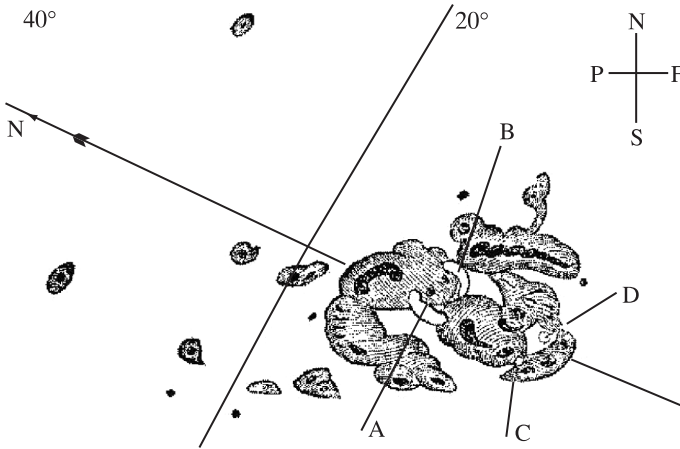
Рис. 1. Зарисовка «белой» (в интегральном свете) солнечной вспышки 1 сентября 1859 г., сделанная Р. Кэррингтоном А, В, С, Д – узлы «белой» вспышки
