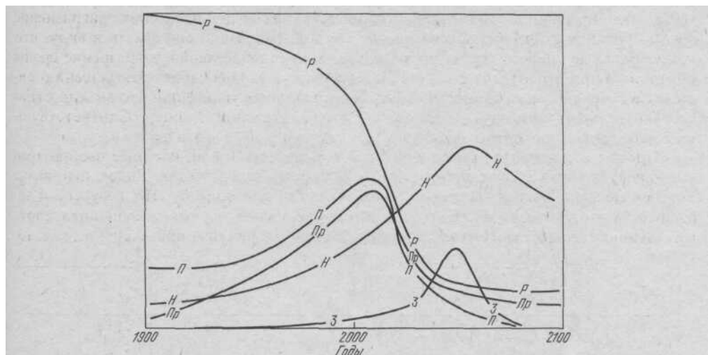
Рис. 111. Стандартная модель мирового развития: P — ресурсы, П — количество пищи на человека в год, H — население земного шара, Pr — промышленное производство, рассчитанное на одного человека, З — загрязнение окружающей среды
