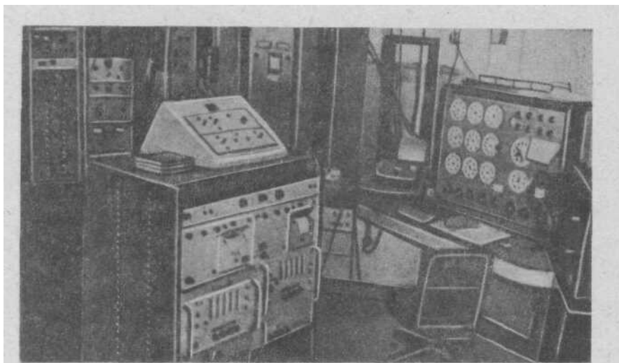
Рис. 96. Приемная аппаратура «ОЗМА»
