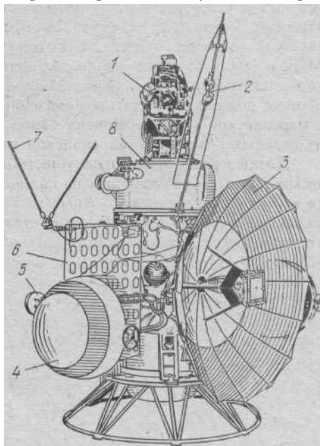
Рис. 61. Автоматическая межпланетная станция «Марс-1»
