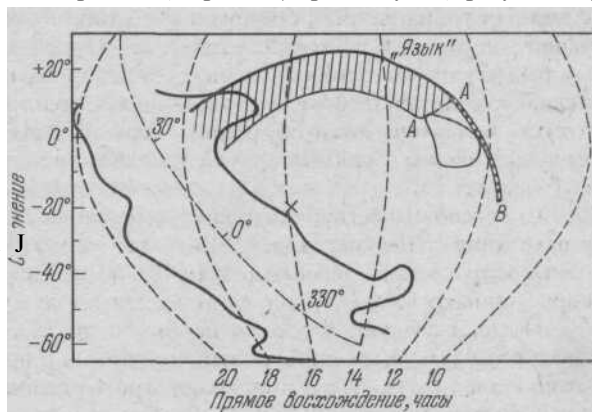
Рис. 28. Изофоты радиоизлучения Галактики (схема)
