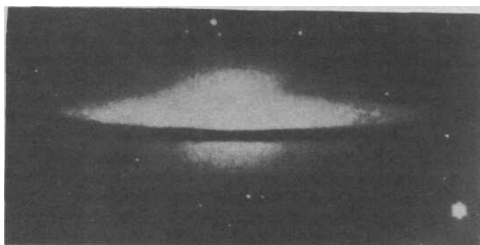
Рис. 6б. Галактика NGC 4594
