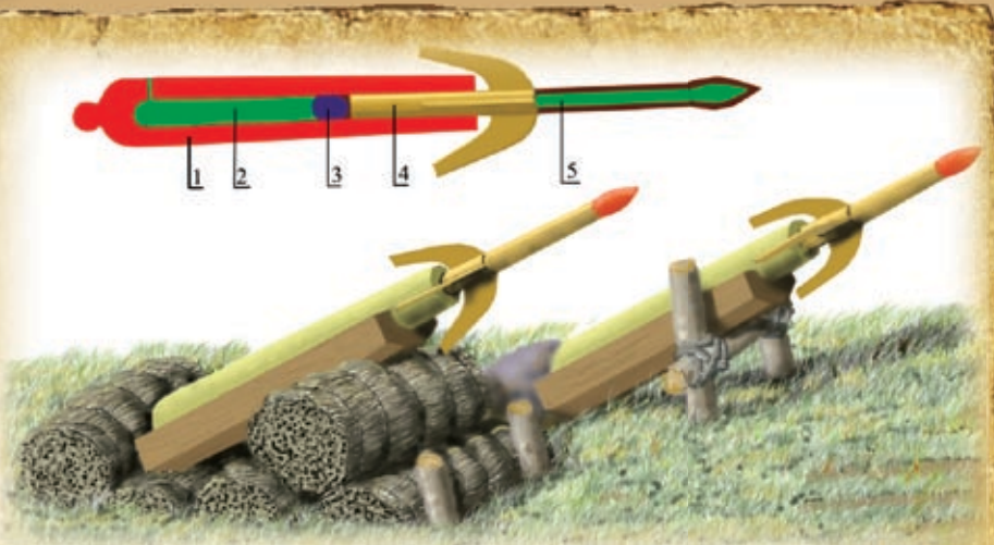
Ракетные установки. 1 — ствол-направляющая; 2 — пороховой заряд оружия; 3 — пых; 4 — ракета; 5 — пороховой заряд ракеты
