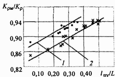
Рис. 29. Зависимость отношения K_{рм}/K_{р} от l_{пу}/L :
