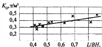
Рис. 46. Зависимость K_D от отношения L/BH
