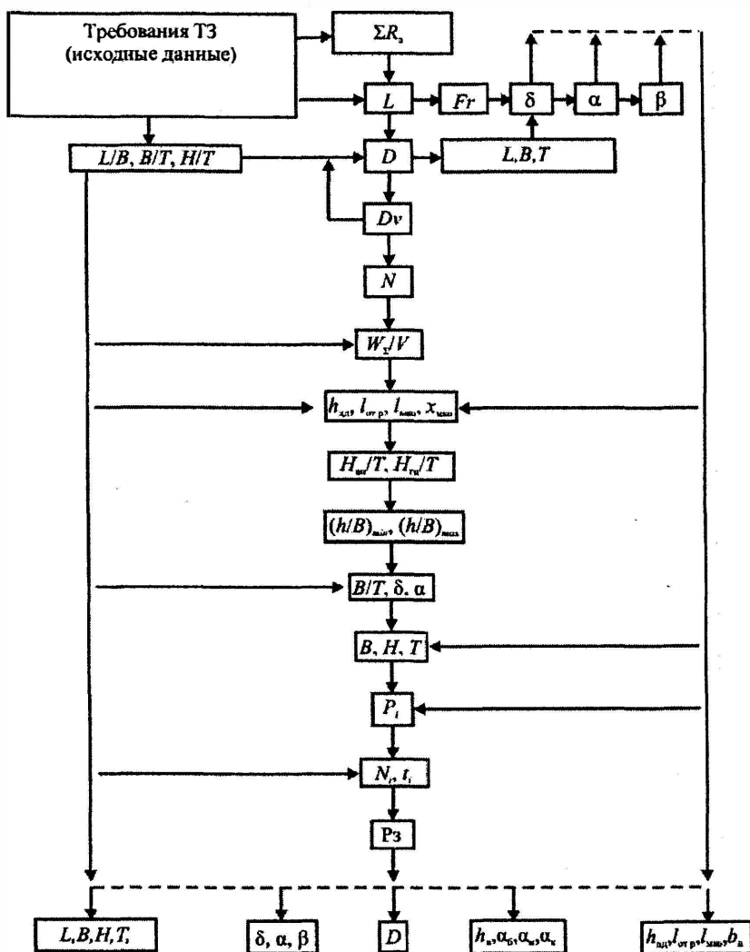
Рис. 45. Последовательность расчета главных размерений КИП
