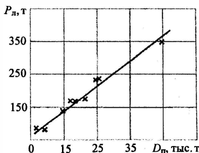
Рис. 35. Зависимость массы льда при обледенении от водоизмещения
