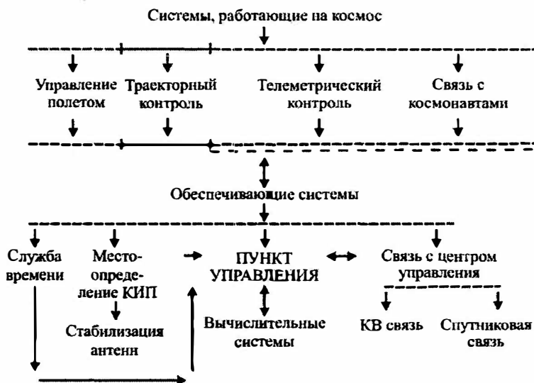
Рис. 2. Структурная схема универсального КИК:
