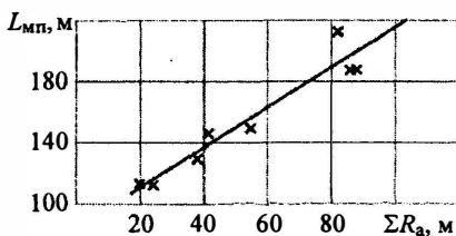
Рис. 47. Зависимость L_{мп} от \Sigma R_a
