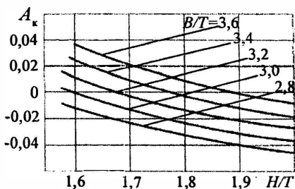
Рис. 34. Графическая интерпретация зависимости (52)
