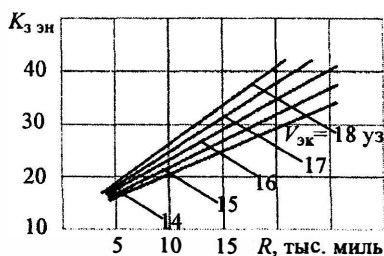
Рис. 23. Графическое представление коэффициента K_{з.эн} при A=120 сут., n_{ж}=300 чел
