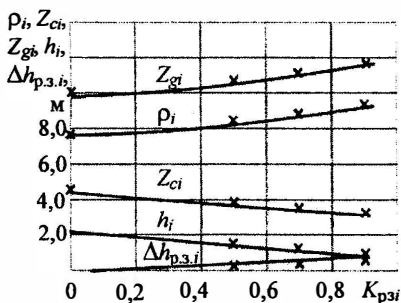
Рис. 33. Результаты расчета элементов остойчивости при различных K_{pi}
