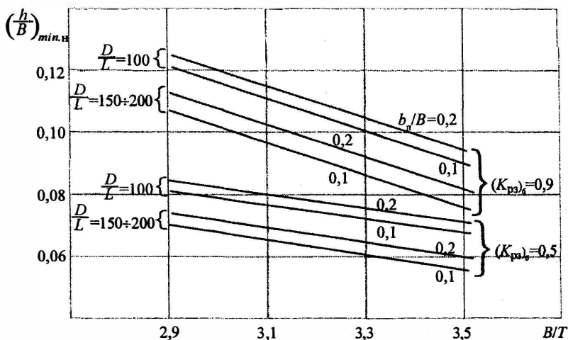
Рис. 42. Зависимость (h/B)_{min} от B/T , (K_{pz})_6 , b_n/B и D/L
