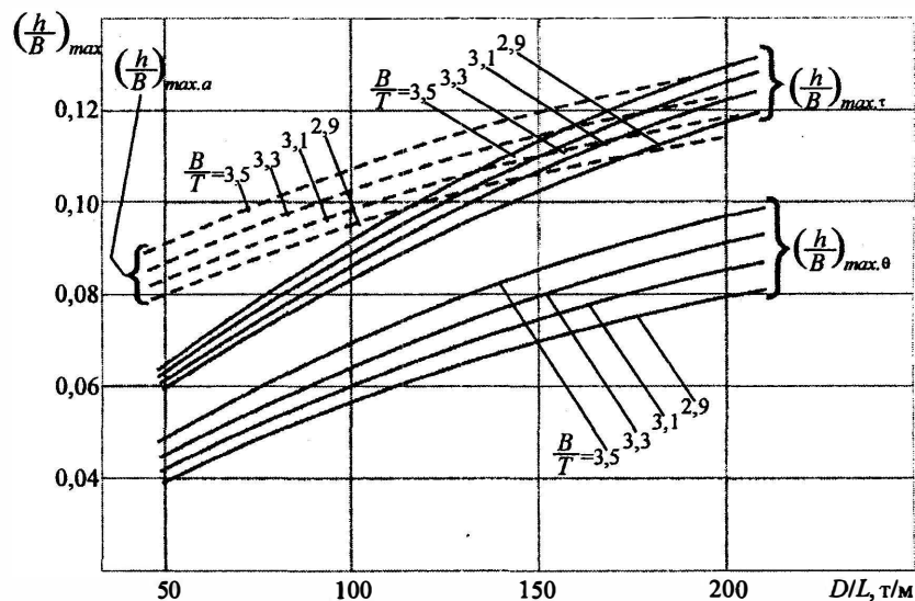
Рис. 43. Графическая интерпретация зависимостей (h/B)_{\max} от D/L и B/T по различным критериям характеристик качки.
