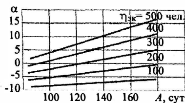
Рис. 24. Поправка к величине K_{з.эн} на отклонение от принятых значений A и n_{ж}
