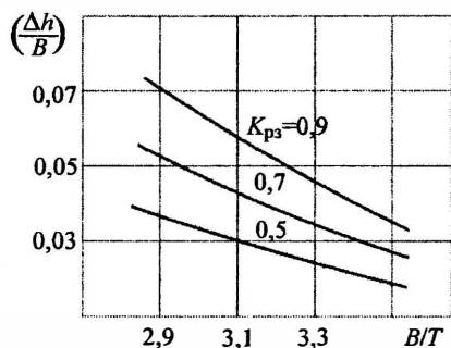
Рис. 37. Графическая интерпретация зависимости (59)
