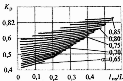
Рис. 30. Графическая интерпретация зависимости (43)
