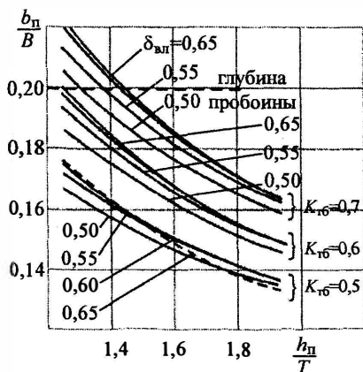
Рис. 18. Графическая интерпретация зависимости b_{\text{п}}/B
