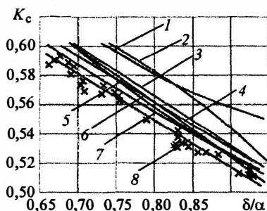
Рис. 31. Графическая интерпретация зависимостей K_c от \delta/\alpha , рекомендованных рядом авторов
