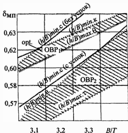
Рис. 49. Совмещенный график элементов и характеристик КИП
