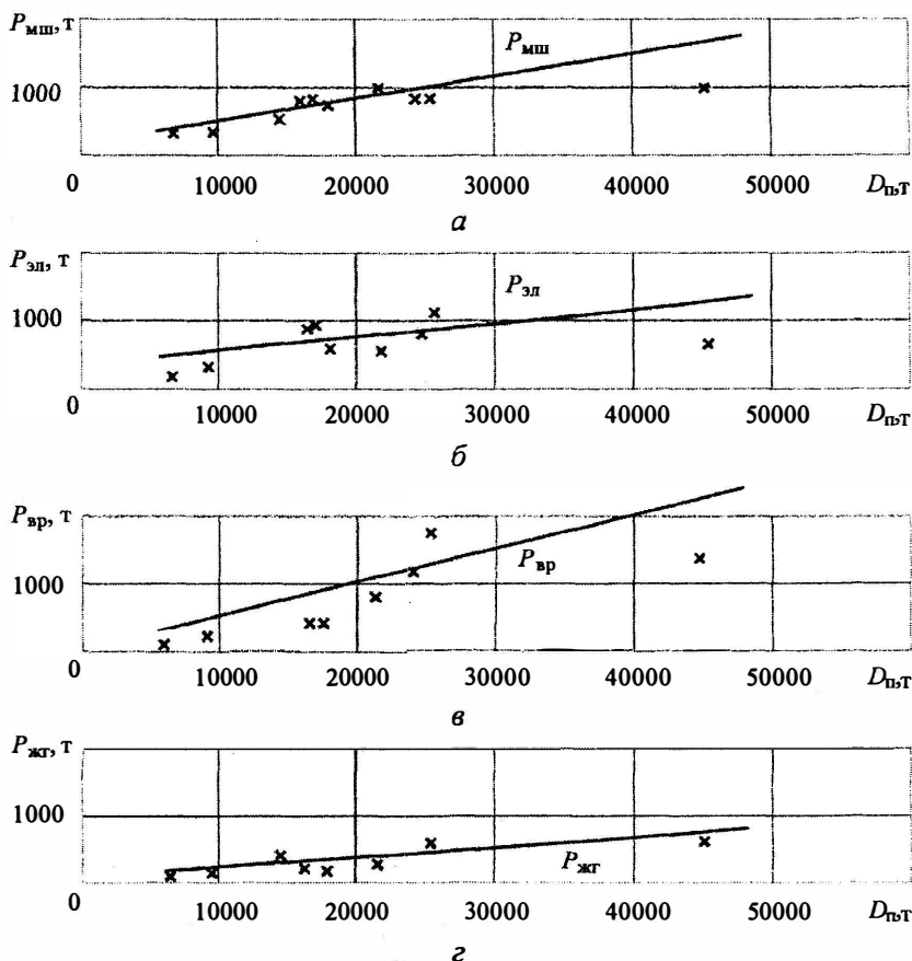
Рис. 22. Зависимость масс по разделам от полного водоизмещения: а – ЭУ, P_{мш} ; б – ЭЭС- P_{эл} ; в – вооружения, P_{вр} ; г – жидких грузов, P_{жг}
