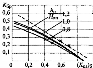
Рис. 26. Графическая интерпретация зависимости (27) и фактические значения K_{6p} для отдельных КИП
