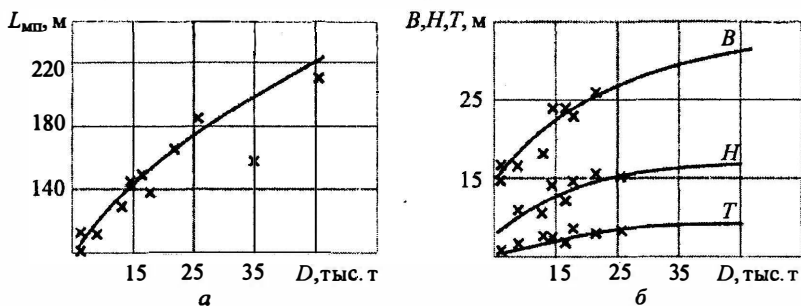
Рис. 48. Связь главных размерений отечественных КИП с водоизмещением: L(a) ; T, H_{\text{вп}}, B(b)
