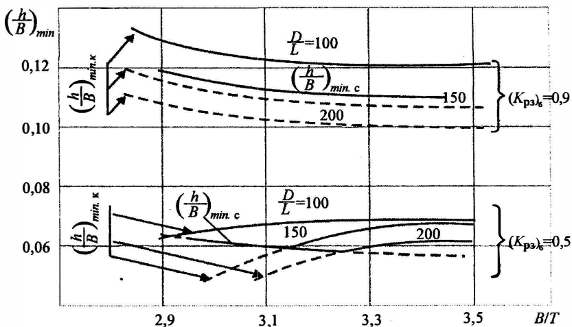
Рис. 41. Зависимость (h/B)_{\min c} и (h/B)_{\min k} от B/T и (K_{pz})_6
