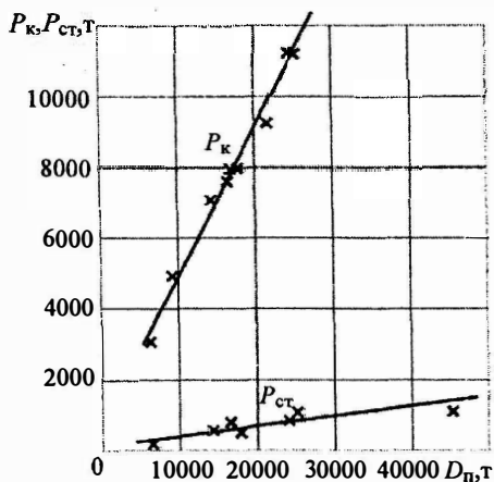
Рис. 21. Зависимость массы корпуса P_k и массы систем P_{ст} от полного водоизмещения D_n
